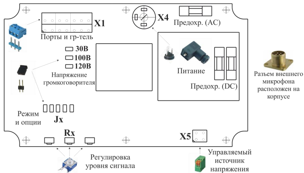
Рисунок 5 – Размещение элементов на плате прибора Тема-АС11.хх-xxx-х65
