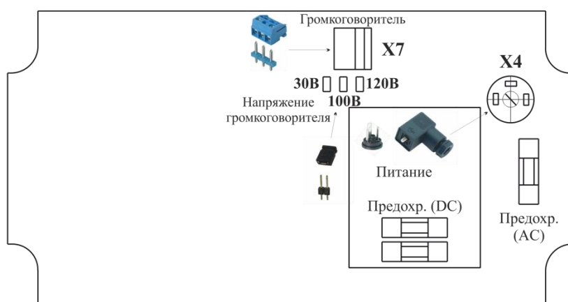
Рисунок 7 – Размещение элементов на нижней плате прибора Тема-A81.62-m65
