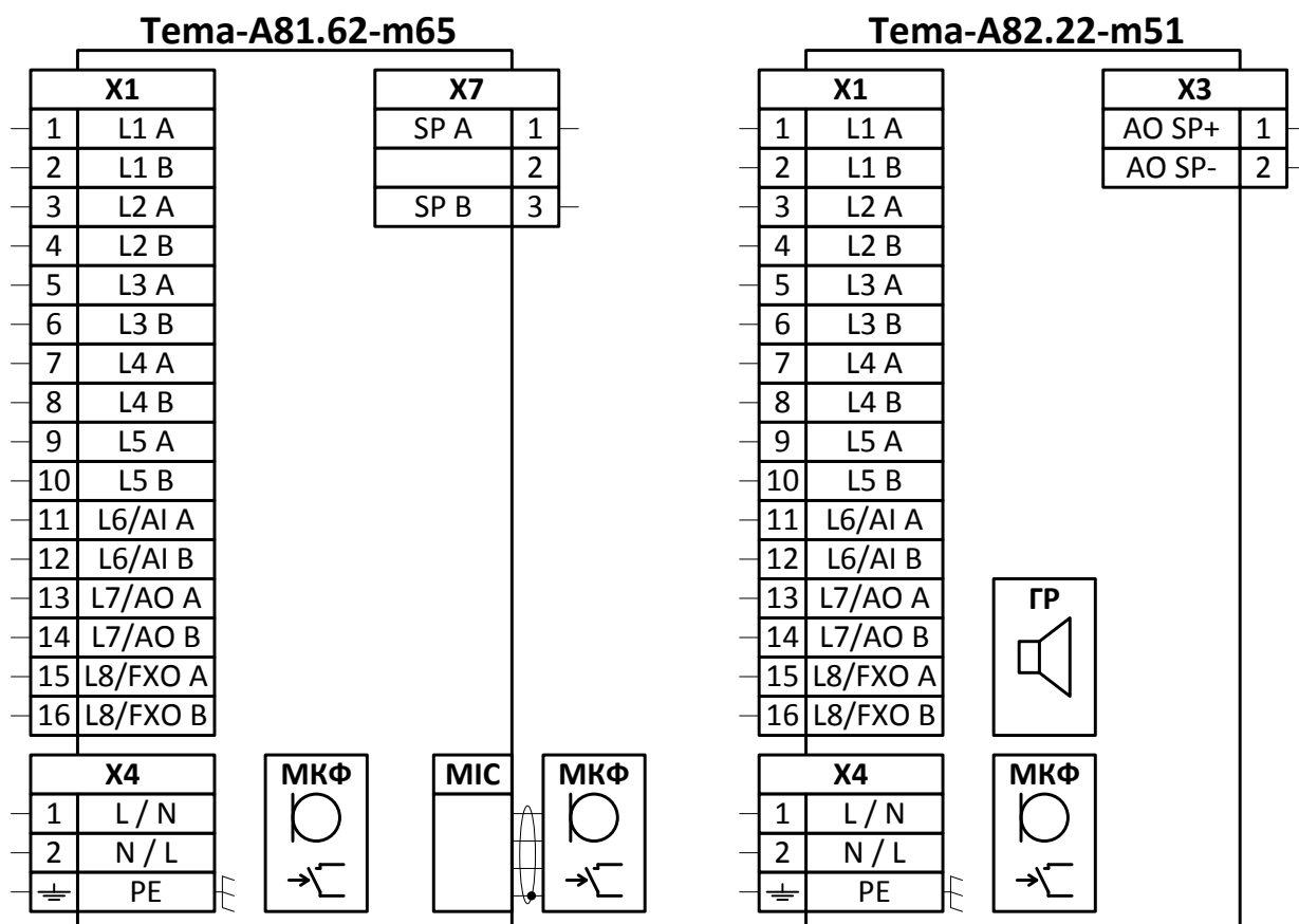
Рисунок 3 – Условное графическое обозначение прибора Тема-A8x.x2
