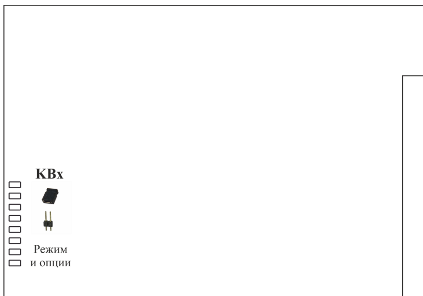
Рисунок 5 – Размещение элементов на верхней плате прибора Тема-A82.22-m51
