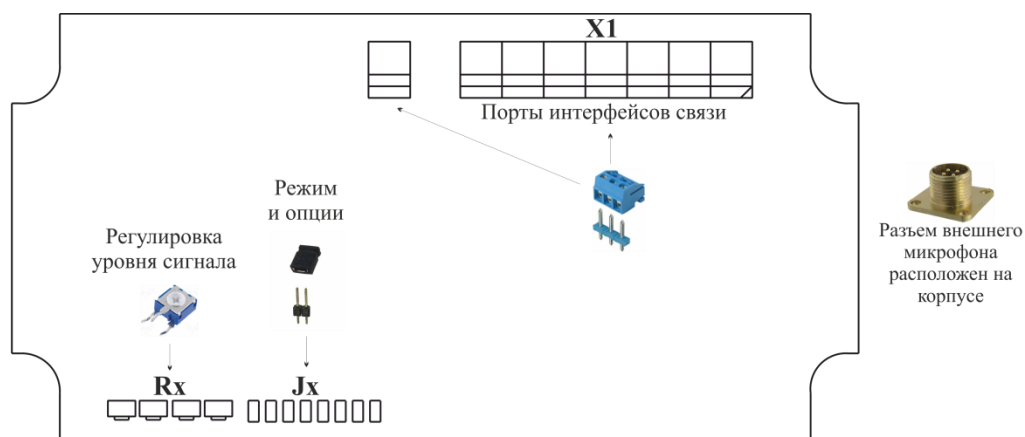
Рисунок 6 – Размещение элементов на верхней плате прибора Тема-A81.62-m65
