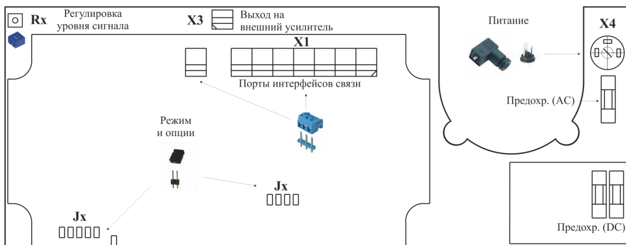
Рисунок 4 – Размещение элементов на нижней плате прибора Тема-A82.22-m51
