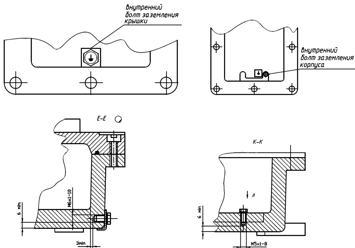
Рисунок Б.4 – Дополнительная информация по средствам заземления корпуса
