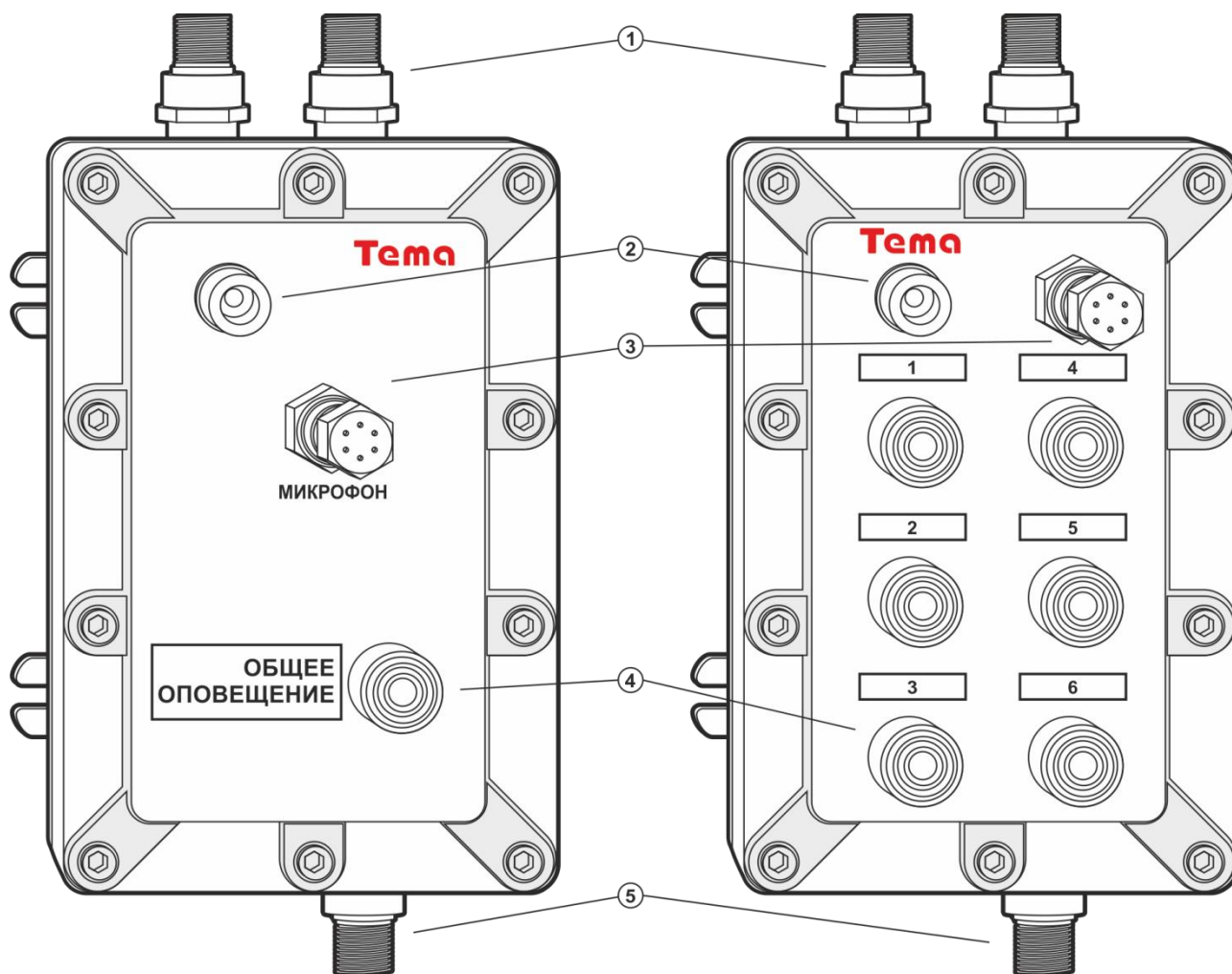
Рисунок 2 – Обобщенный внешний вид модели взрывозащищенного исполнения
