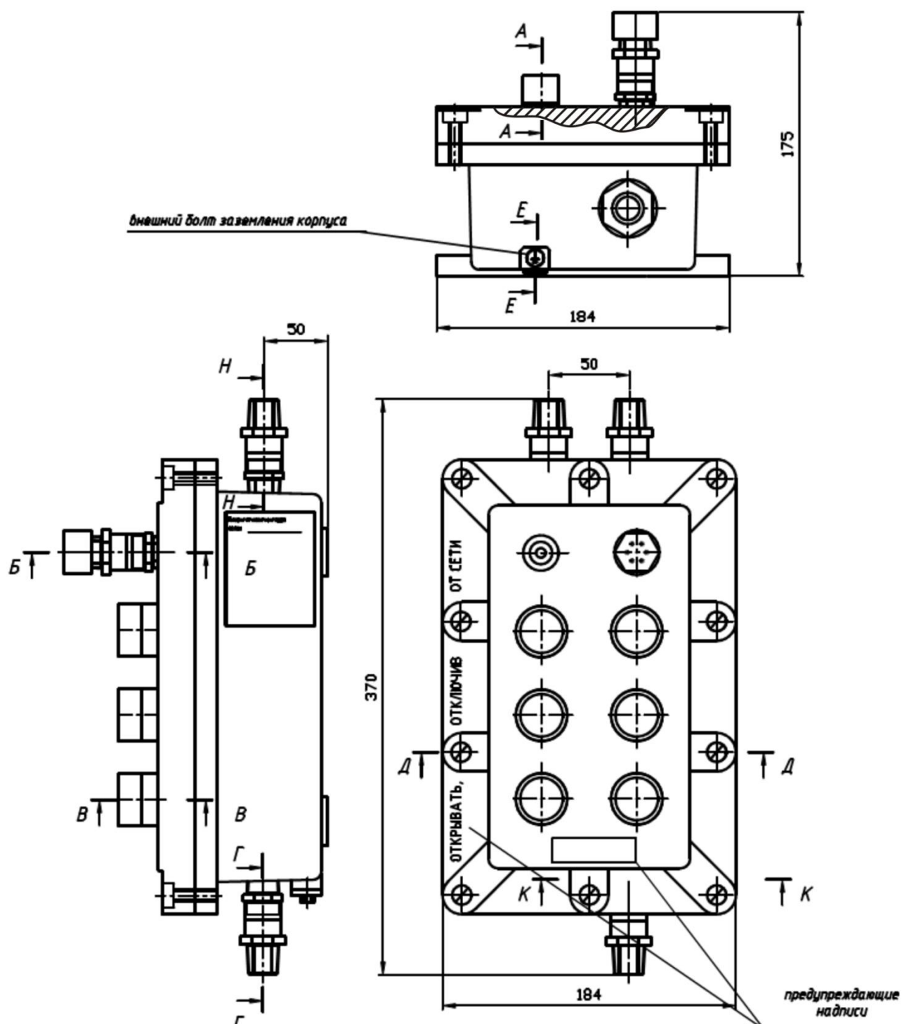
Рисунок Б.2 – Внешний вид взрывозащищенной модели с шестью кнопками
