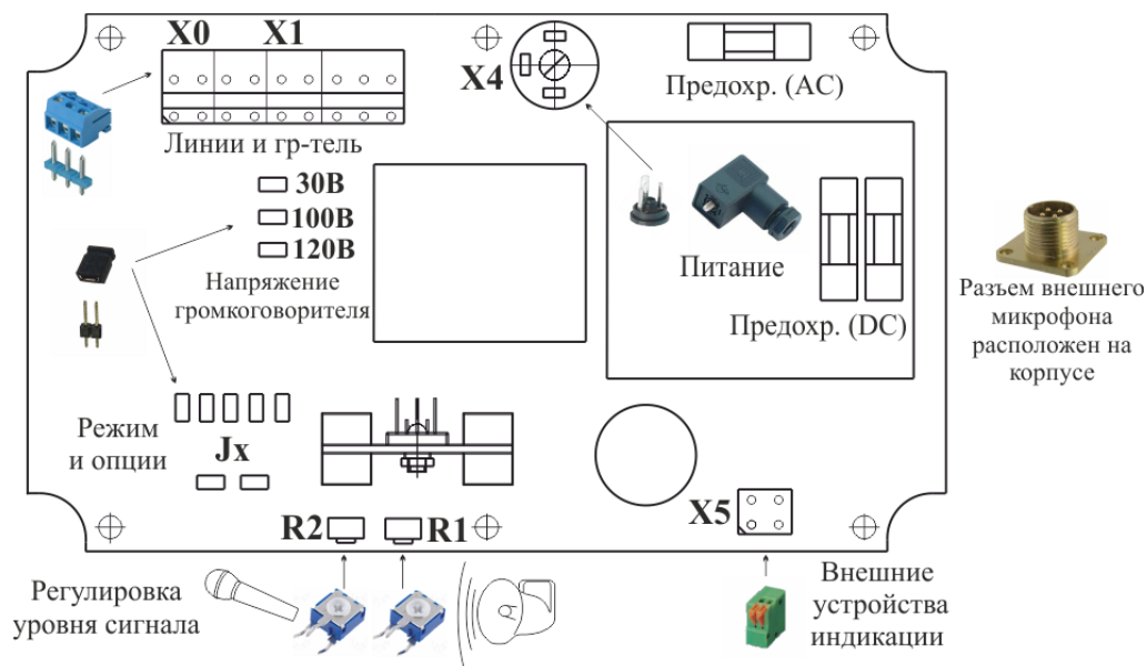
Рисунок 6 – Размещение элементов на плате прибора
