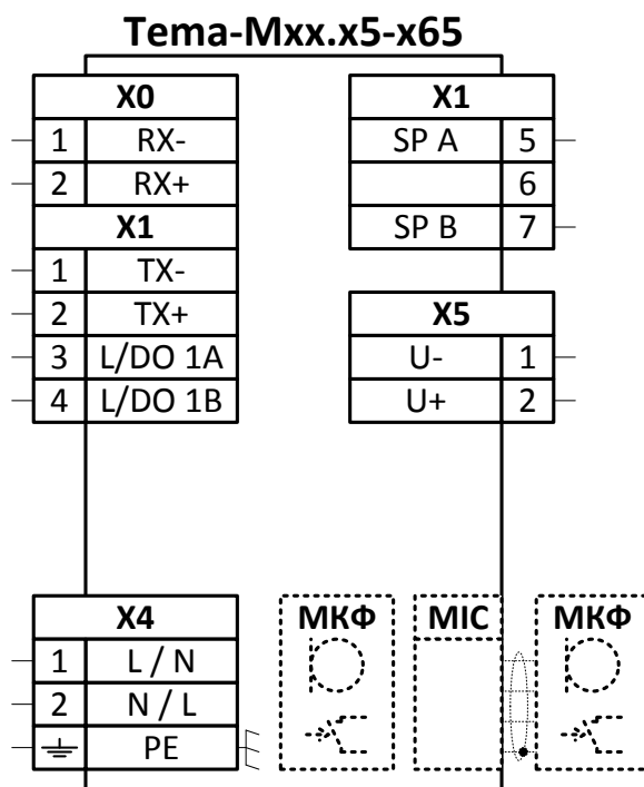
Рисунок 5 – Условное графическое обозначение прибора Тема-Мхх.х5-ххх-х65
