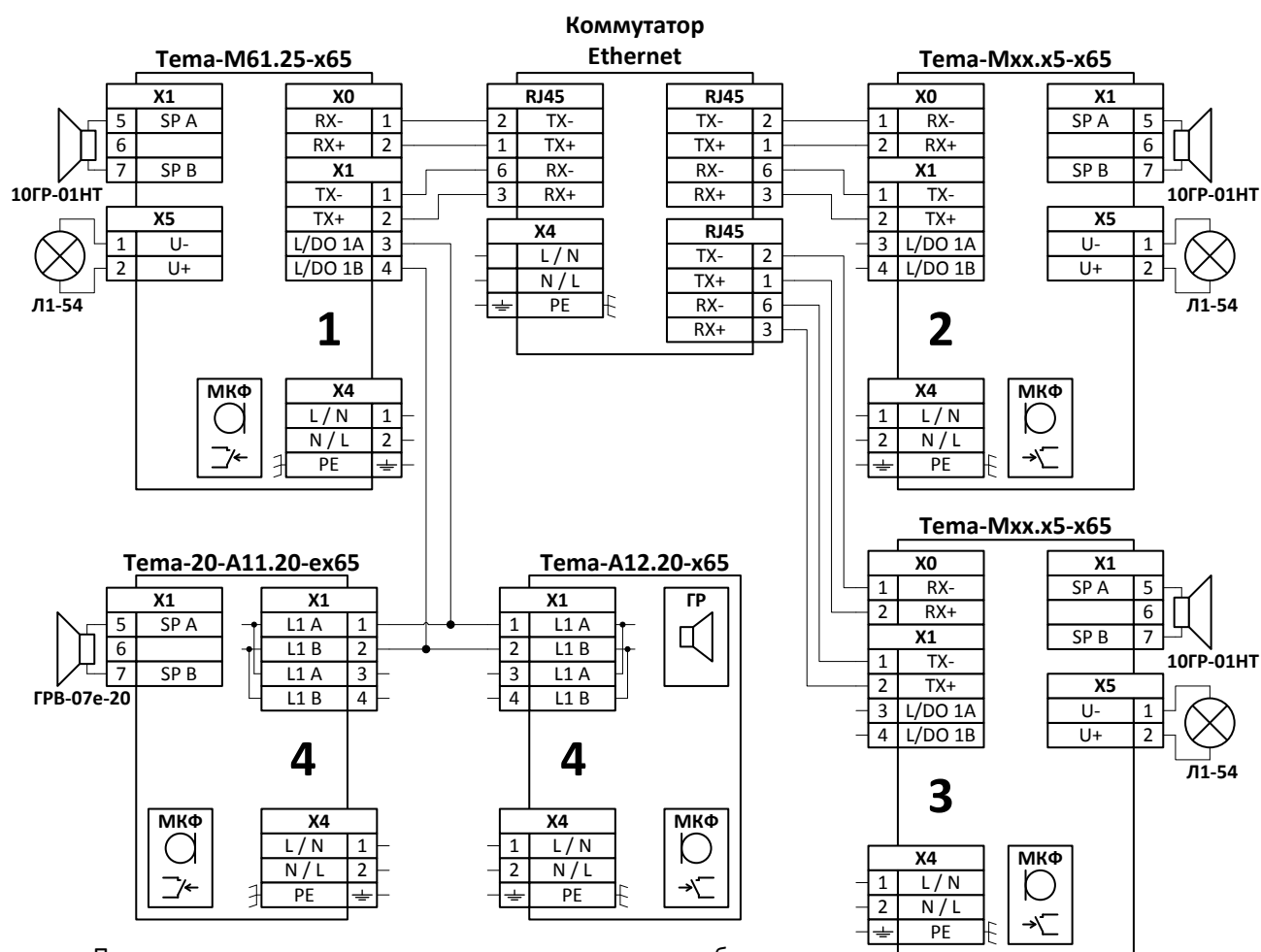
Рисунок 7 – Пример схемы избирательной громкоговорящей связи
