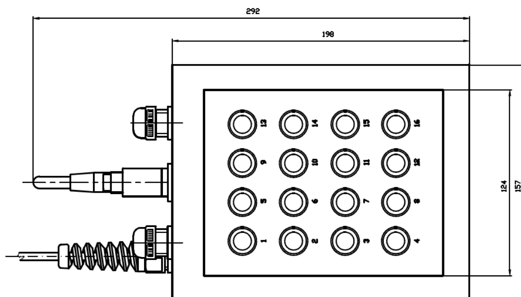
Рисунок А.3 – Габаритные размеры приборов Тема в настольном исполнении
