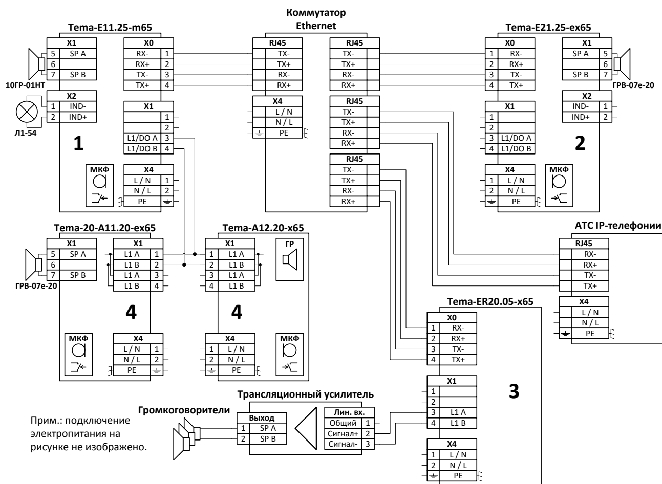
Рисунок 6 – Пример схемы системы избирательной громкоговорящей связи
