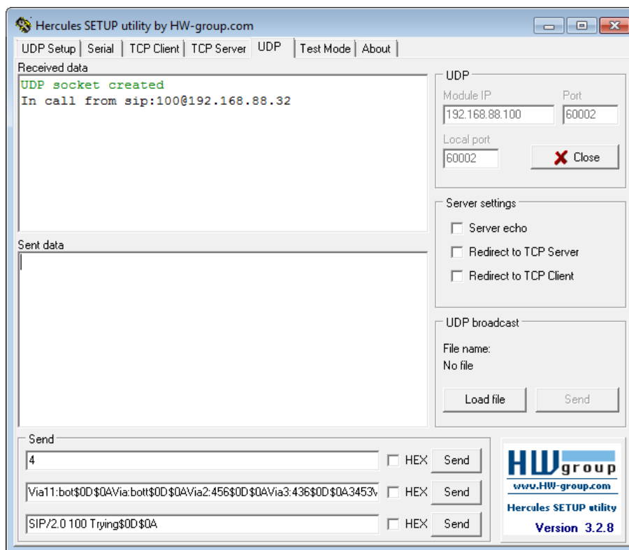
Рисунок 14 – Пример диагностического сообщения при наличии входящего вызова
