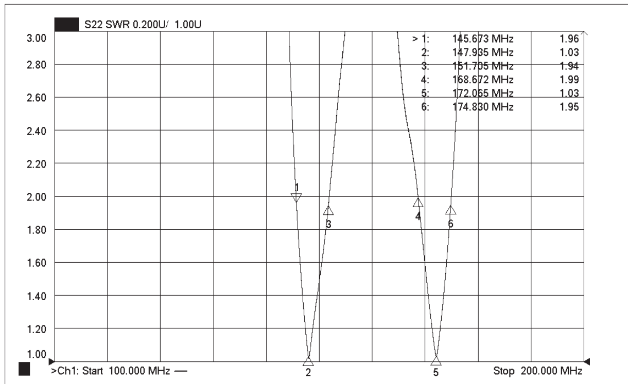
График КСВ
