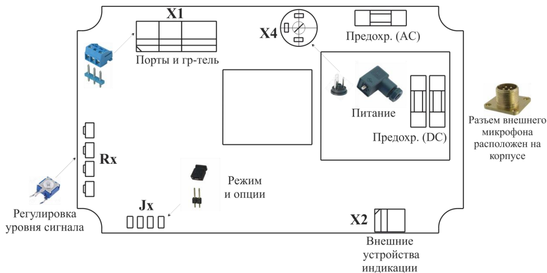
Рисунок 5 – Размещение элементов на плате прибора Тема-АС11.хх-xxx-х65
