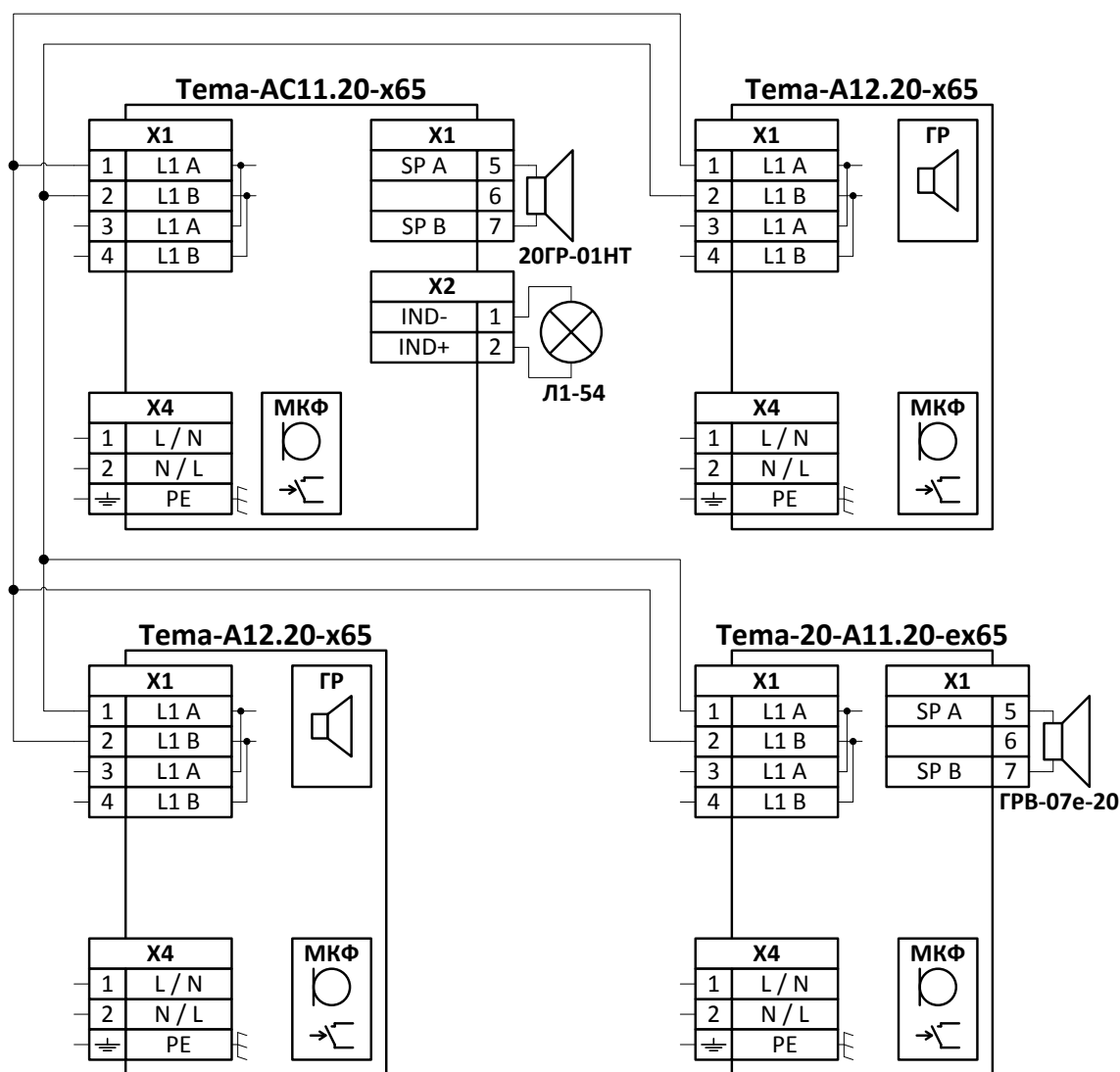
Рисунок 6 – Пример схемы включения «Один говорит – все слышит»
