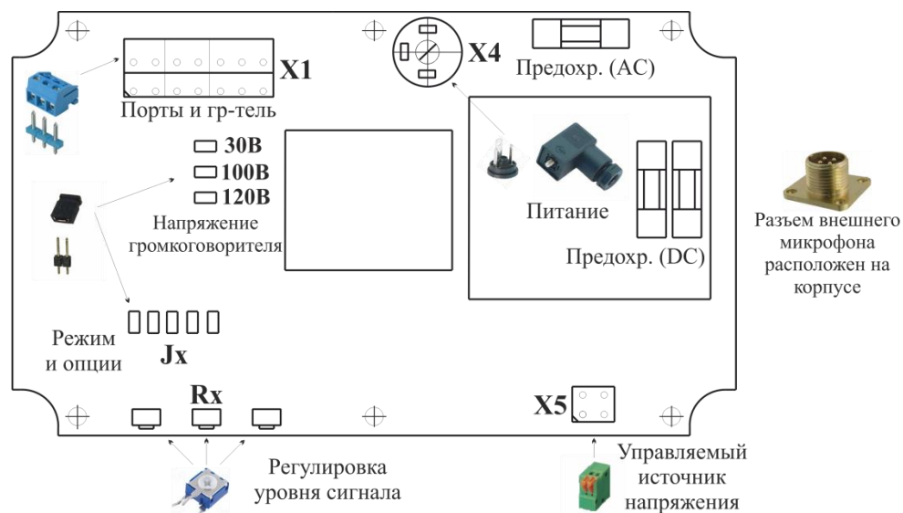
Рисунок 5 – Размещение элементов на плате прибора Тема-АС11.xx-xxx-x65
