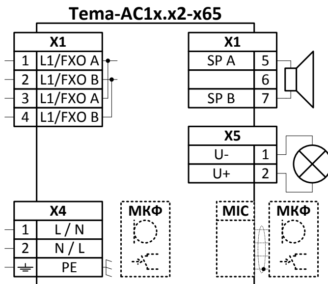
Рисунок 4 – Условное графическое обозначение прибора Тема-АС11.x2-xxx-x65
