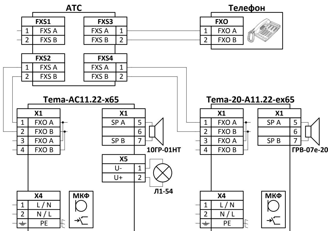
Рисунок 6 – Пример схемы подключения к АТС
