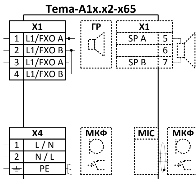
Рисунок 4 – Условное графическое обозначение прибора Тема-хх-A1х.х2-ххх-х65
