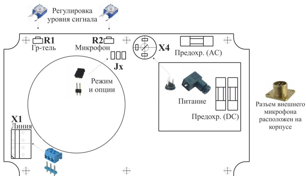
Рисунок 6 – Размещение элементов на плате прибора Тема-A12.x2-xxx-x65
