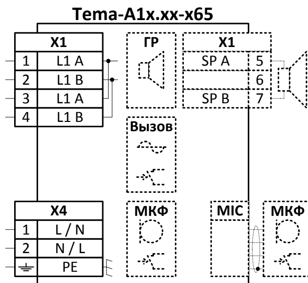
Рисунок 4 – Условное графическое обозначение прибора Тема-хх-A1х.хх-ххх-х65
