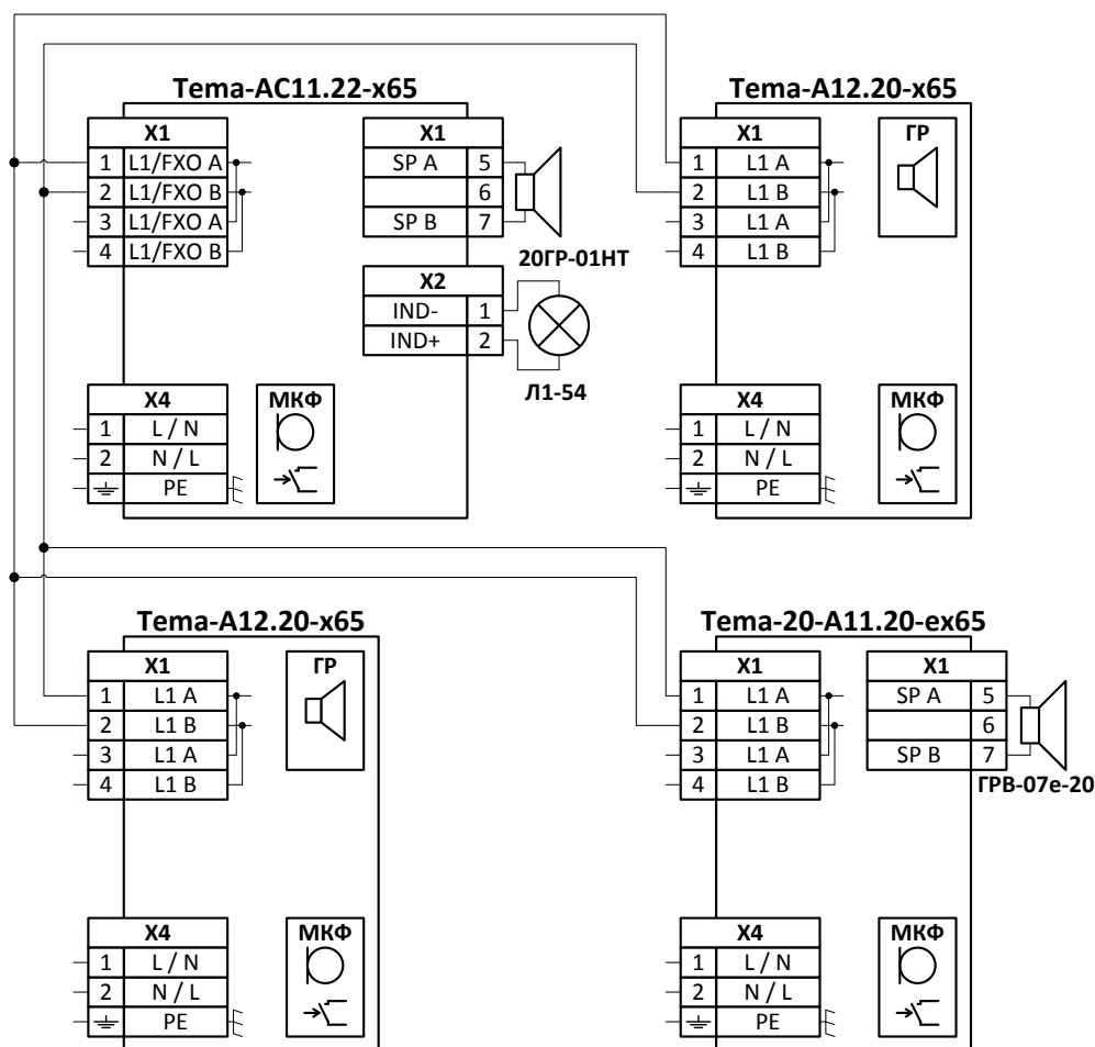
Рисунок 7 – Пример схемы включения «Один говорит – все слышат»
