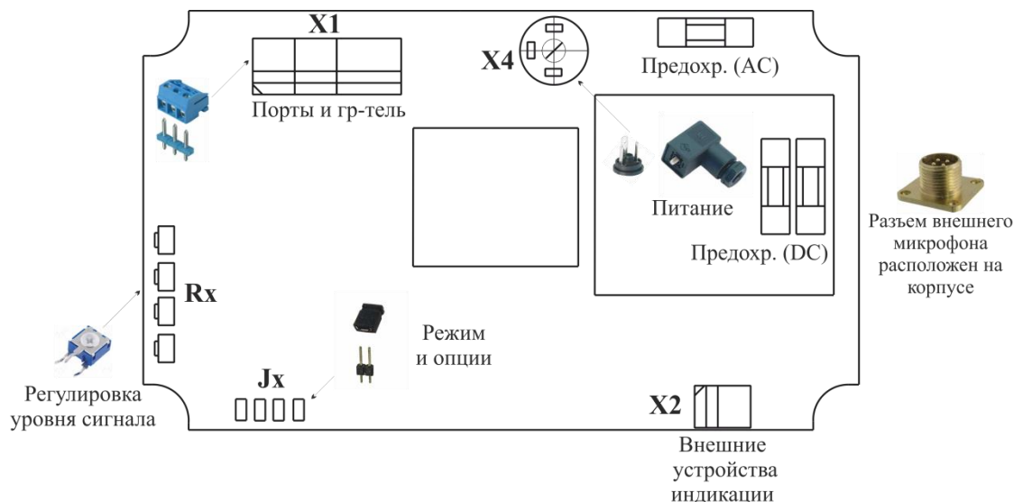
Рисунок 5 – Размещение элементов на плате прибора Тема-АС11.xx-xxx-x65
