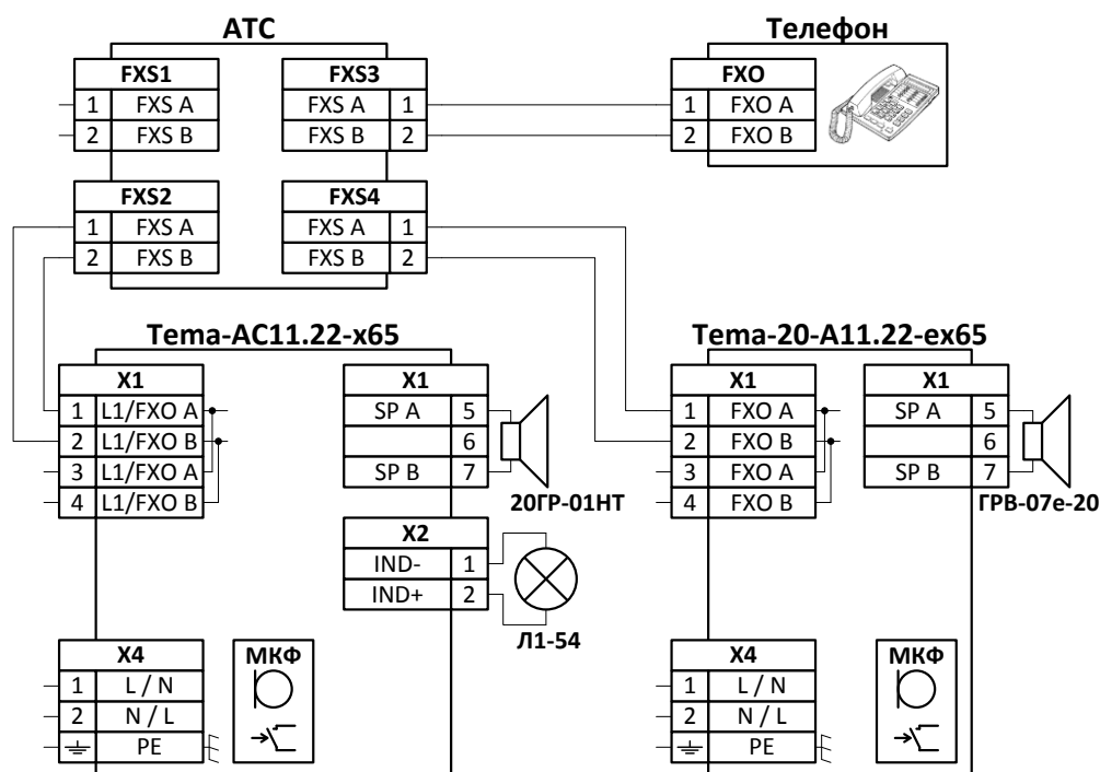
Рисунок 6 – Пример схемы подключения к АТС
